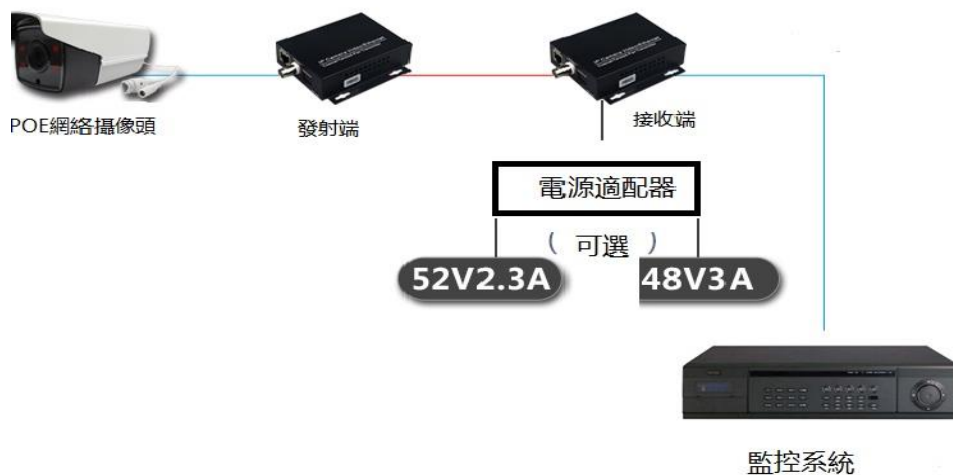
POE模式連接示意圖
