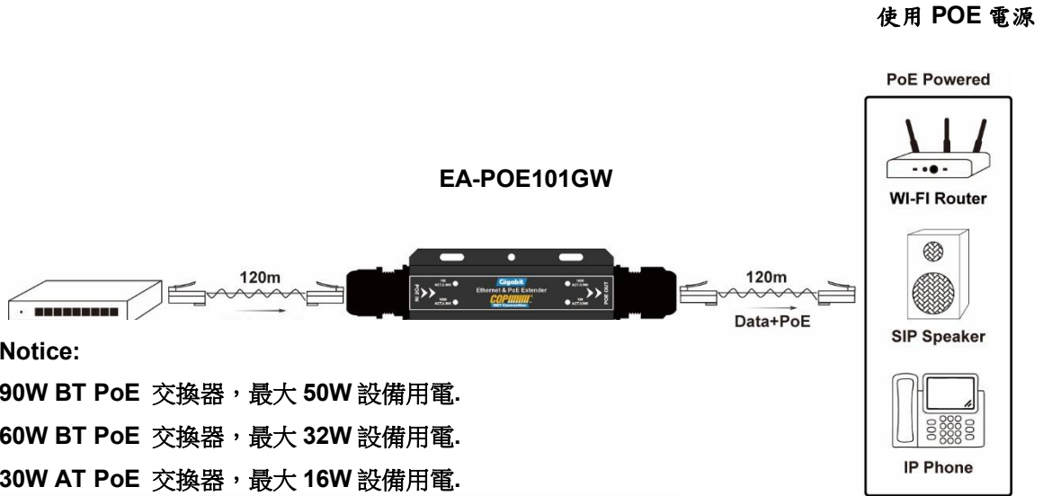
EA-POE101GW 應用圖 1: 中繼 PoE 電源和網路資料至 IP 裝置
