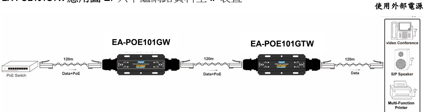
EA-POE101GTW 應用圖 2: 只中繼網路資料至 IP 裝置
