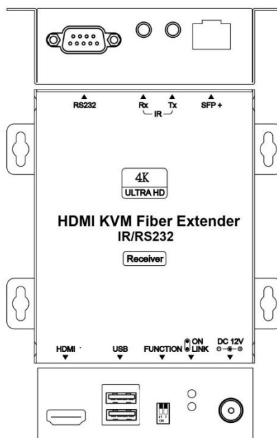
HE01FR-4K6G
